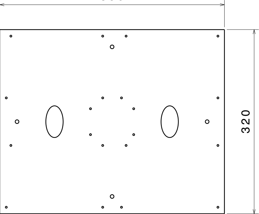
Vue de face Echelle : 1:4
